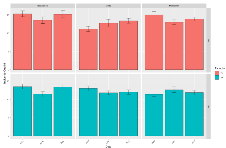
Figure 4. Indice de qualité des huîtres diploïdes (rouge), triploïdes (bleu) de mai 2021 à juillet 2021 en grossissement sur les zones de Bouzigues, Mèze et Marseillan.
